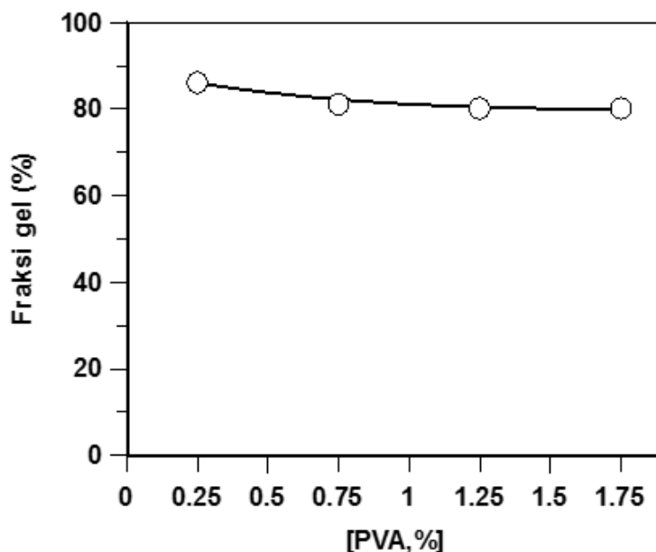
Gambar 8. Hubungan konsentrasi PVA vs. fraksi gel hidrogel kopolimer(kalium akrilat)- g-PVA hasil iradiasi 10 kGy
