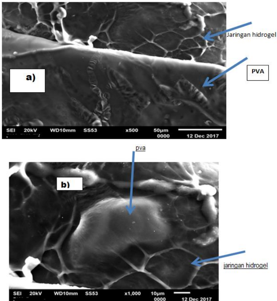
Gambar 2. Foto SEM hidrogel kopoli (kaliumakrilat)-g-PVA hasil iradiasi 10 kGy pada perbesaran a) 500 dan b) 1000 kali
