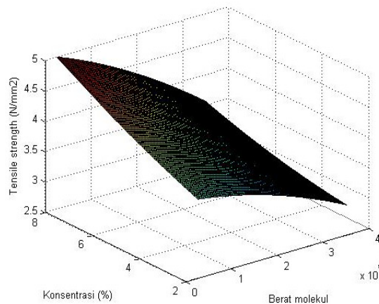
Gambar 1. Pengaruh berat molekul dan konsentrasi kitosan terhadap kekuatan tarik kertas daur ulang
