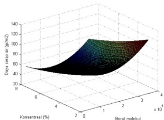
Gambar 2. Berat molekul dan konsentrasi kitosan terhadap daya serap air kertas daur ulang
